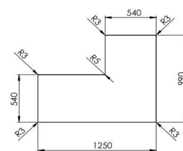
Saison-Funkenschutzplatte 41/6361.2901
