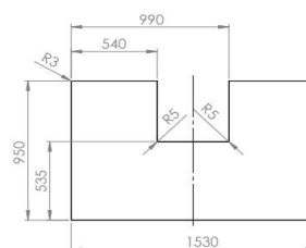
Saison-Funkenschutzplatte 41/6461.2901
