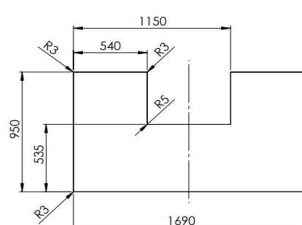
Plaque de protection en verre 41/6161.2901
