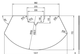
Saison-Funkenschutzplatte 23/2290.2914
