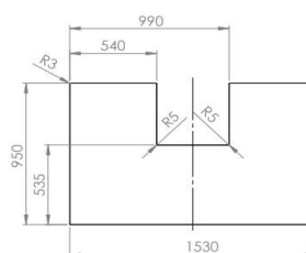
Plaque de protection en verre 41/6461.2901
