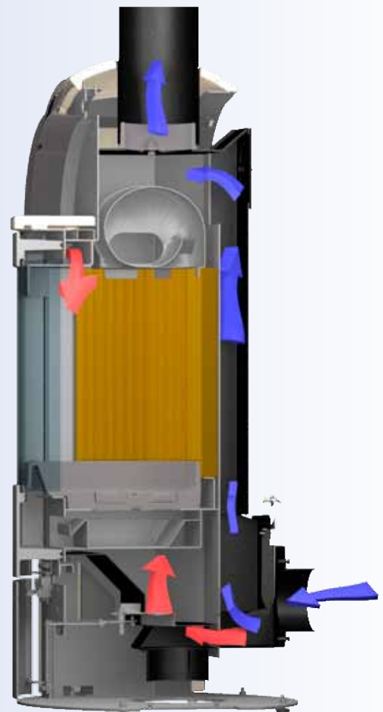
Unterdruck im Feuerraum > 20 Pa Nebenluftklappe beginnt zu öffnen
